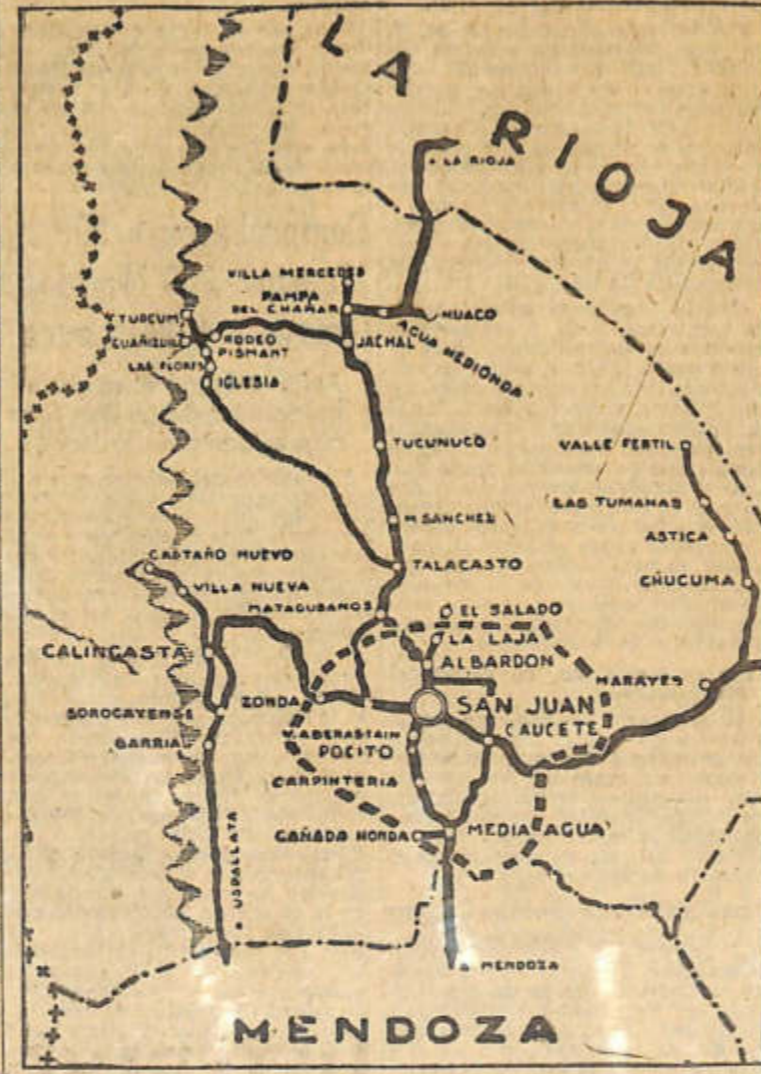
La línea gruesa cortada comprende la zona de plena acción del terremoto
