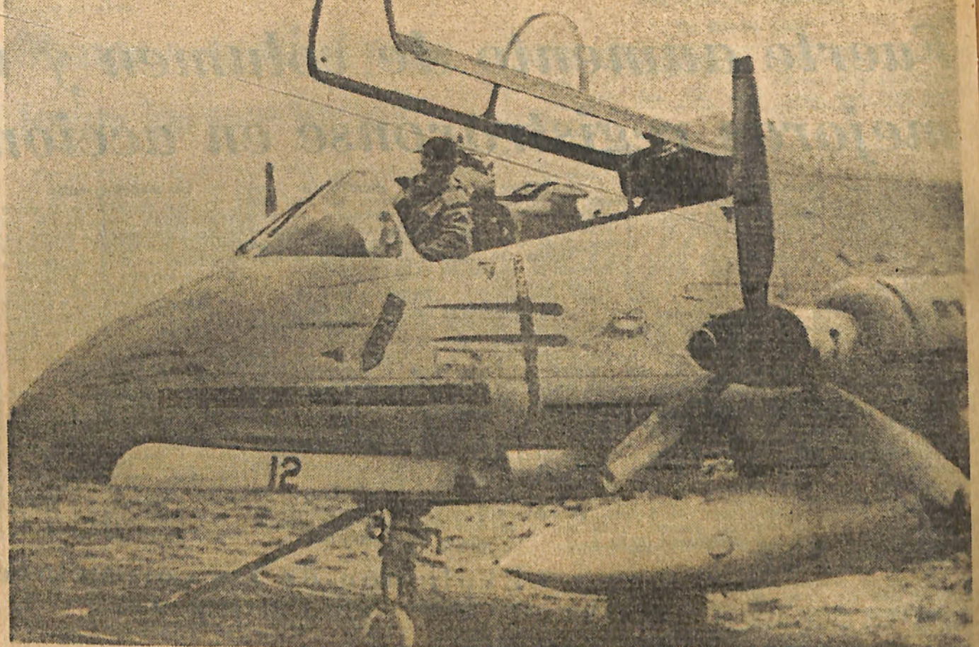
En una base aérea del sur argentino, un piloto militar comprueba el funcionamiento de su avión de combate Pucará
